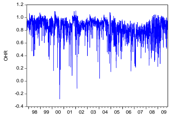
BEKK:BRSP_BRFU
